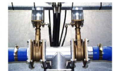
Teilbreitenschaltung rechts/links mit zwei pneumatischen Schieber
