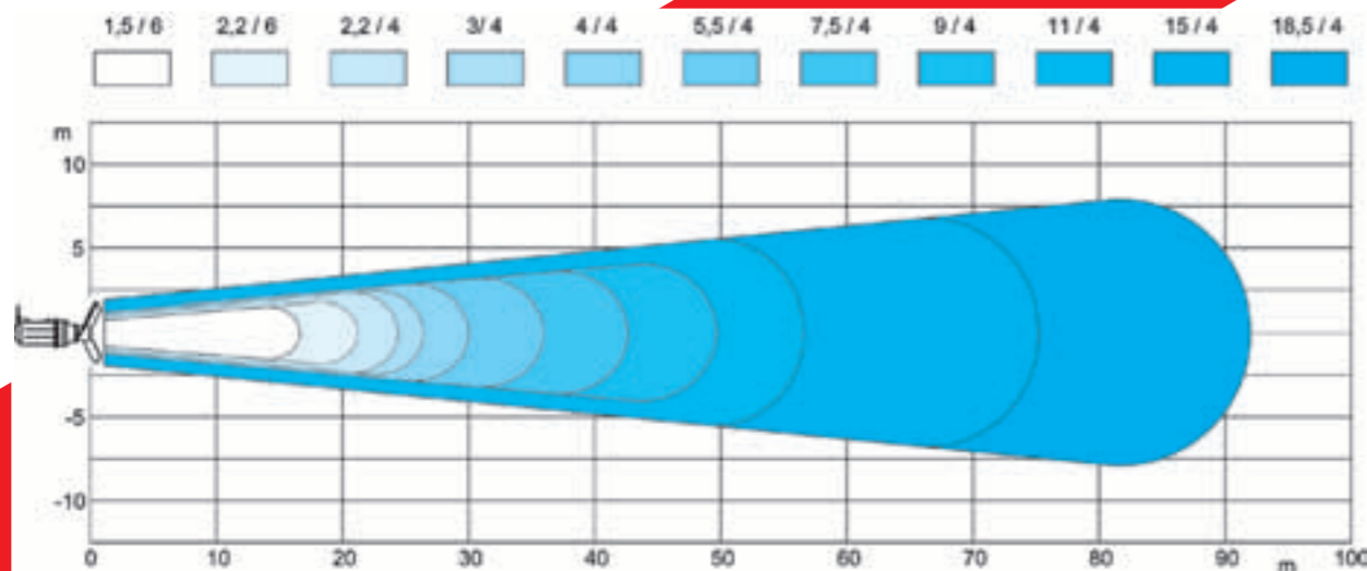
Rührleistung in Wasser bei v=0,3 m/s
